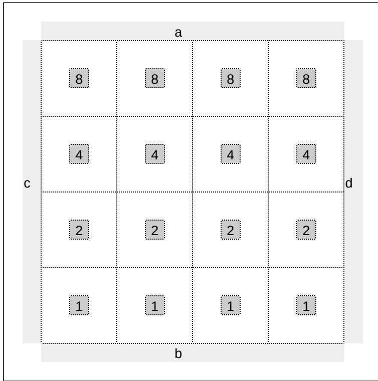
Grundplatte für die LED's und das Gitter
